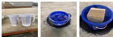
Gambar 3. Pengujian daya apung bata ringan CLC
