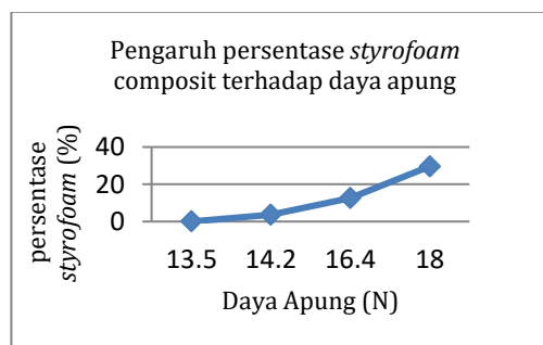
Grafik 1. Pengaruh persentase styrofoam terhadap daya apung.
