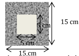
Gambar 2. Desain benda uji dengan penambahan styrofoam 3,70%
